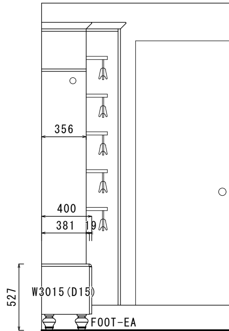
ベンチ部分断面
